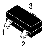
SOT23(TO-236)
